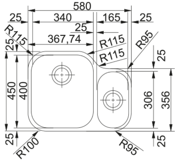
Мойка AMX 160, 580x450 мм, без крыла, нерж.сталь, 3 1/2", вентиль, короб
