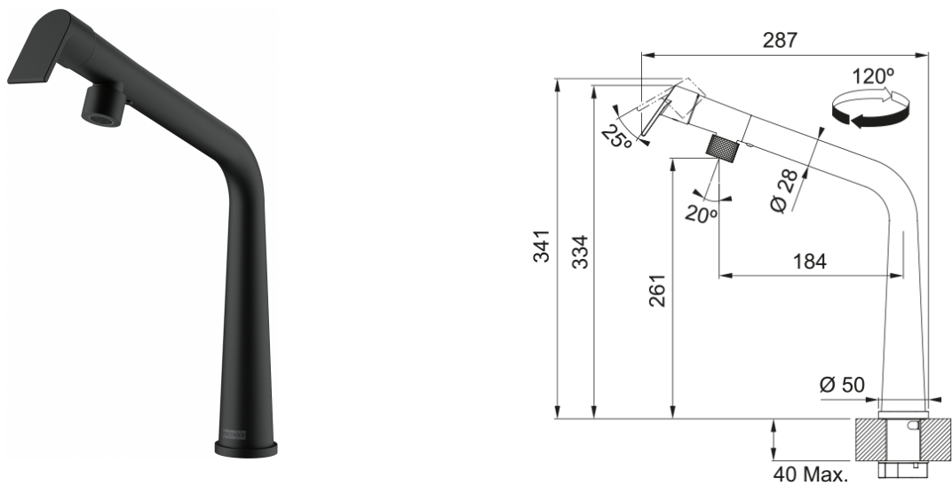
Смеситель Icon с поворотным изливом, черный матовый
