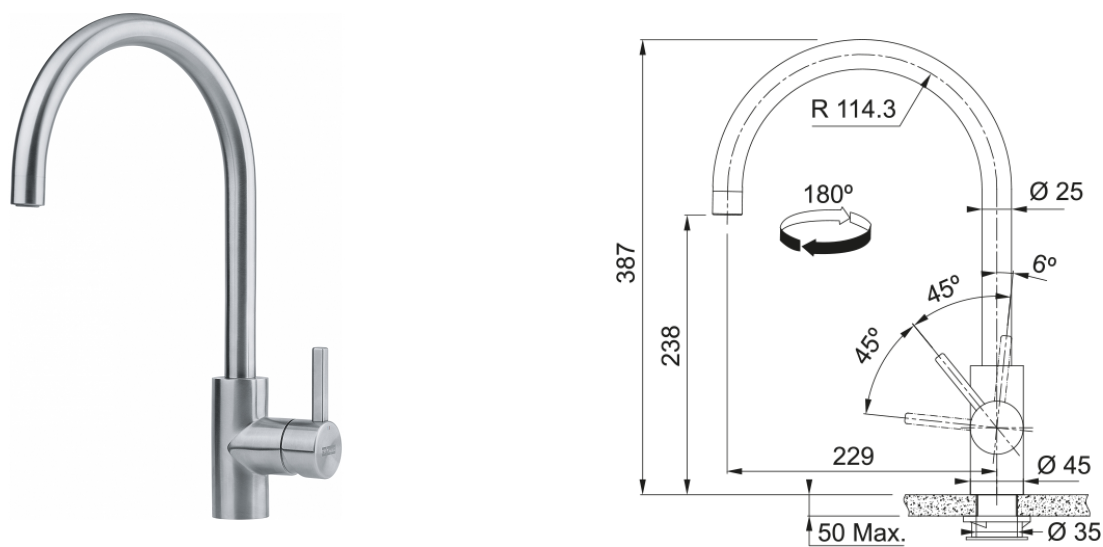
Tap Eos Neo Swivel Side HP SS AU
