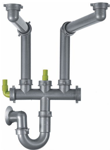
Sifone plastico doppio
