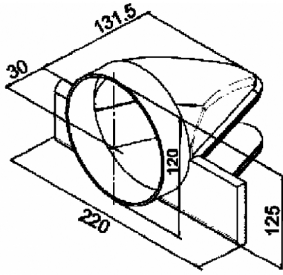
Curva reversibile CRCO 90 Cod. 6098016
