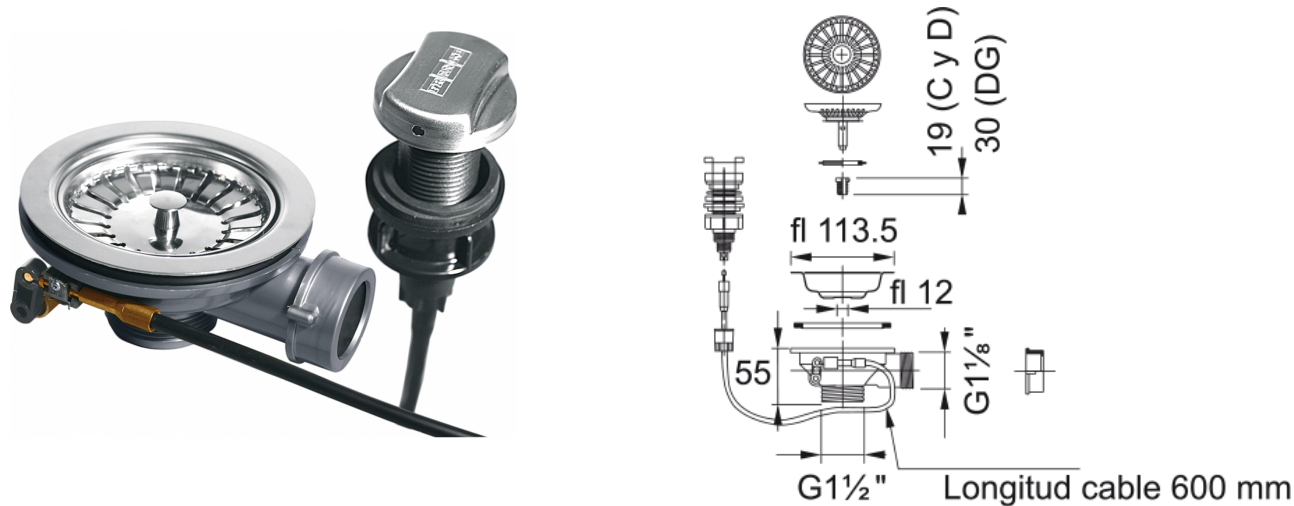
Válvula Automática 3" ½ Mando estándar
