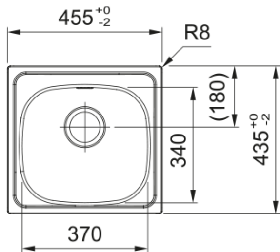
SKN 610-37/44 Edelstahl ungebürstet, Einbau, 1 Becken, 455x435mm, 3 1/2" Stopfenventil
