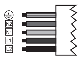
380V - 415V 2N ~
