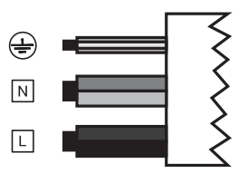
220V - 240V 1N ~
