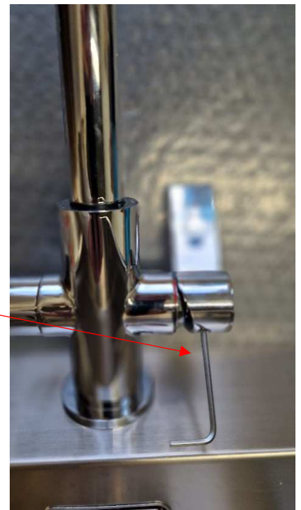
Kuva Kahvan kiristys 2,5mm kuusiokoloavaimella
