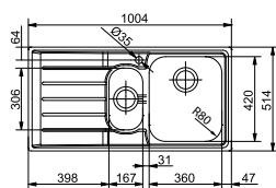
Vlaktbouw / SlimTop
