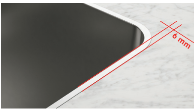
Vlakkouw/SlimTop
