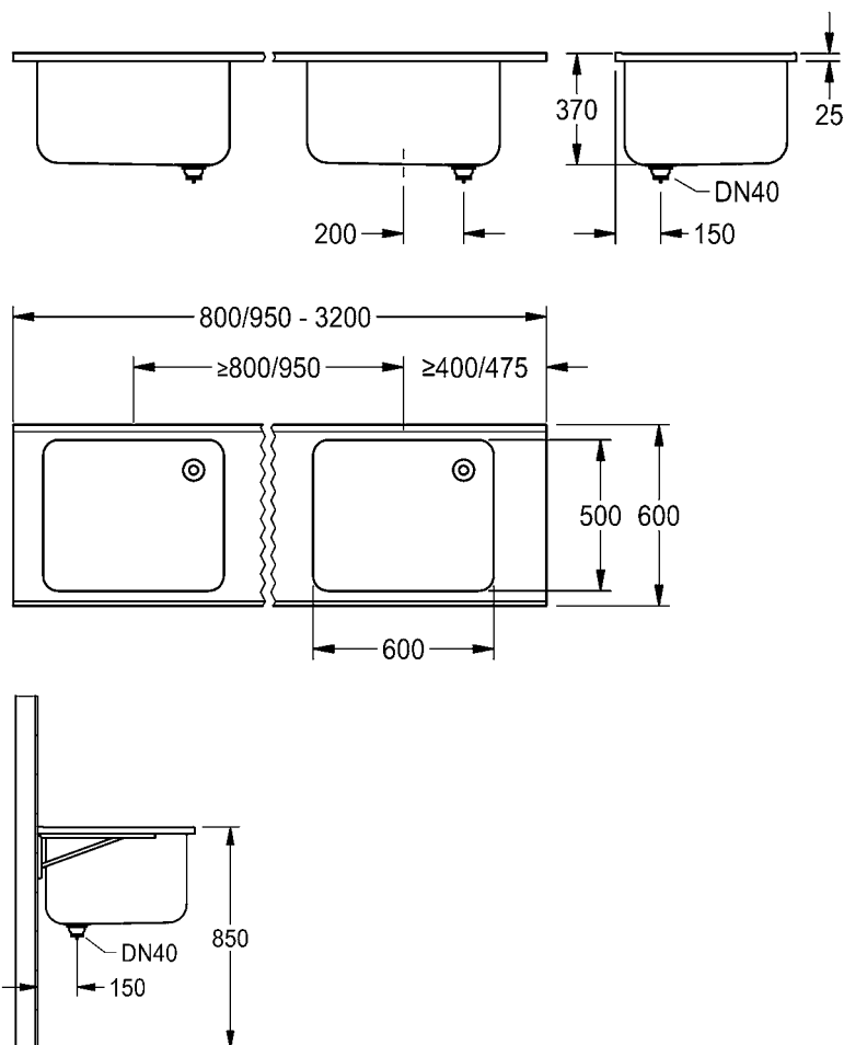
Exemple de bassins polyvalents VARIUSmed avec vasque latérale
