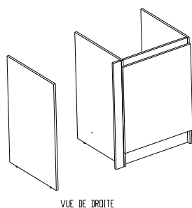
VUE DE DROITE
