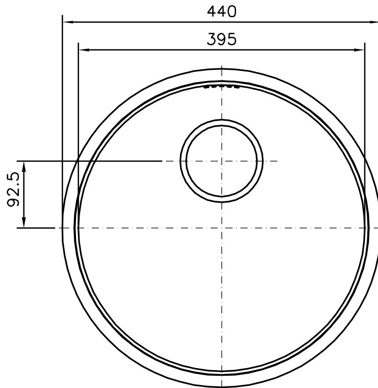
Huullosaukon mitat = altaan ulkomitat
