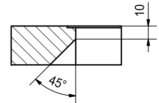
C-C (1 : 2)
