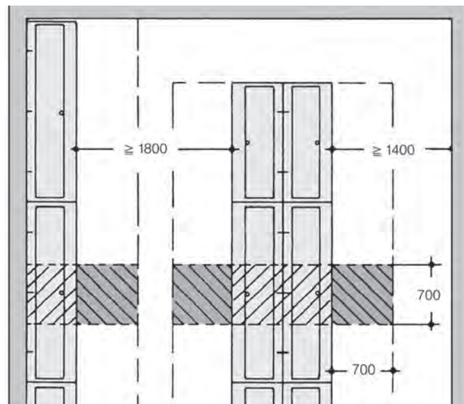
Flächenbedarf für ein- und doppelreihige Reihenwaschanlage
