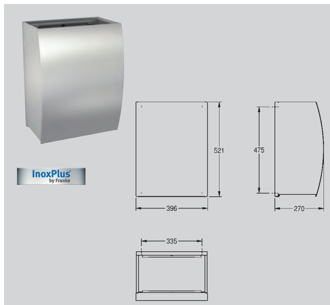
Abbildung und Zeichnung mit Abfallbehälter STRX607.
